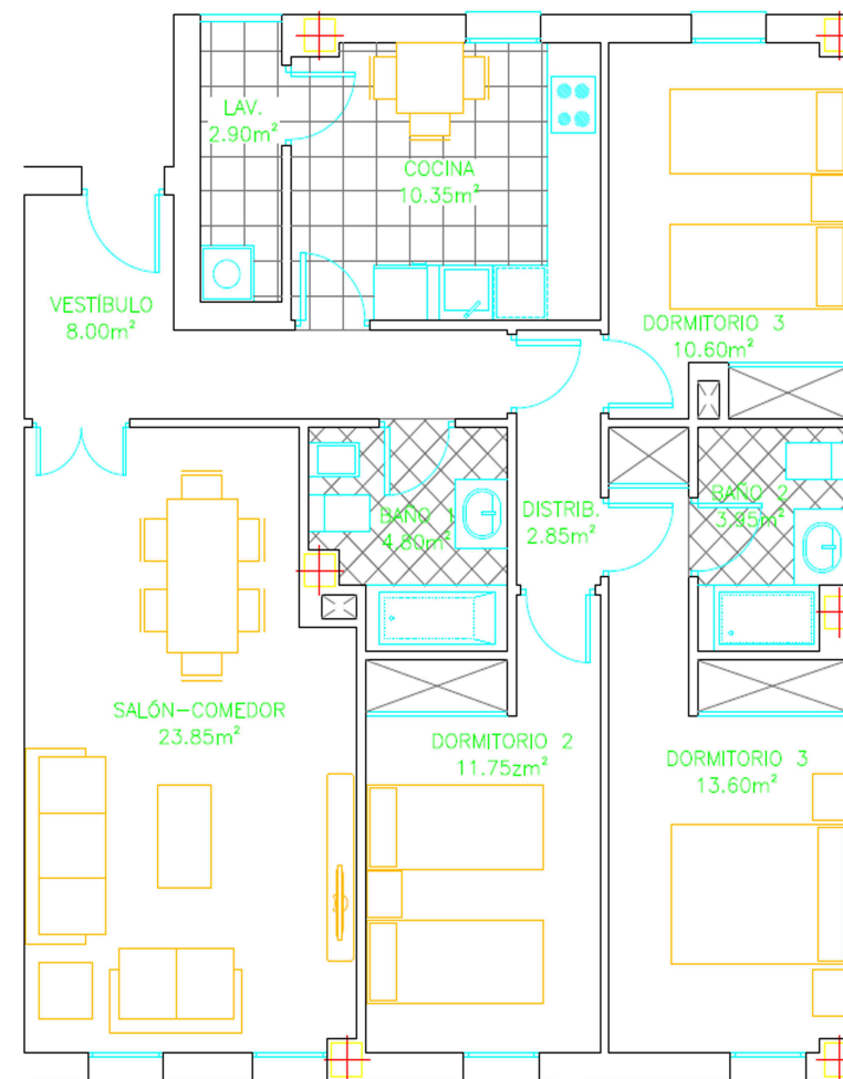
PLANTA DE VIVIENDA
