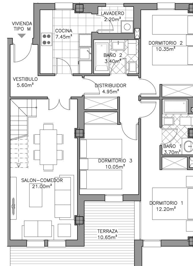
PLANTA DE VIVIENDA
