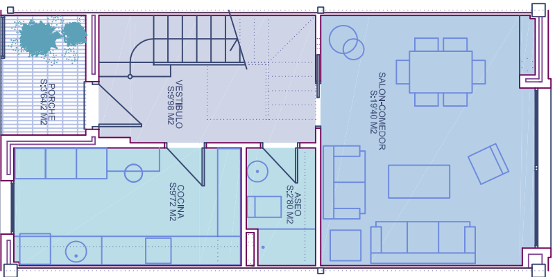
PLANTA BAJA VIVIENDA TIPO DUPLEX SUPERFICIE CONSTRUIDA : 4917 M2 SUPERFICIE UTIL : 4372 M2
